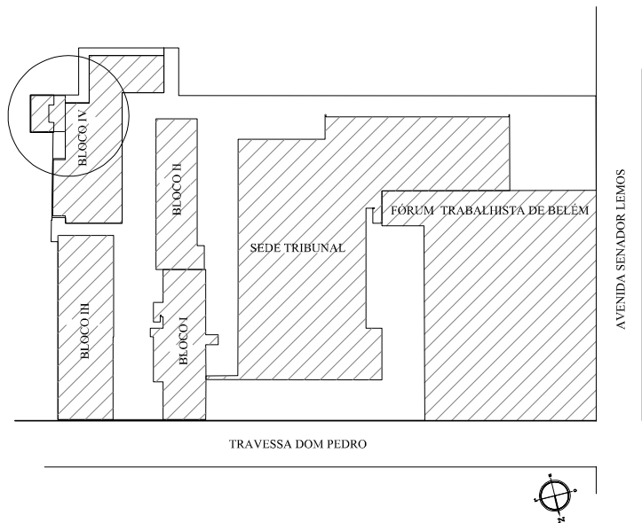
PLANTA DE SITUAÇÃO ESC. 1/500
