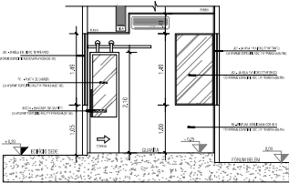
CORTE BB'
