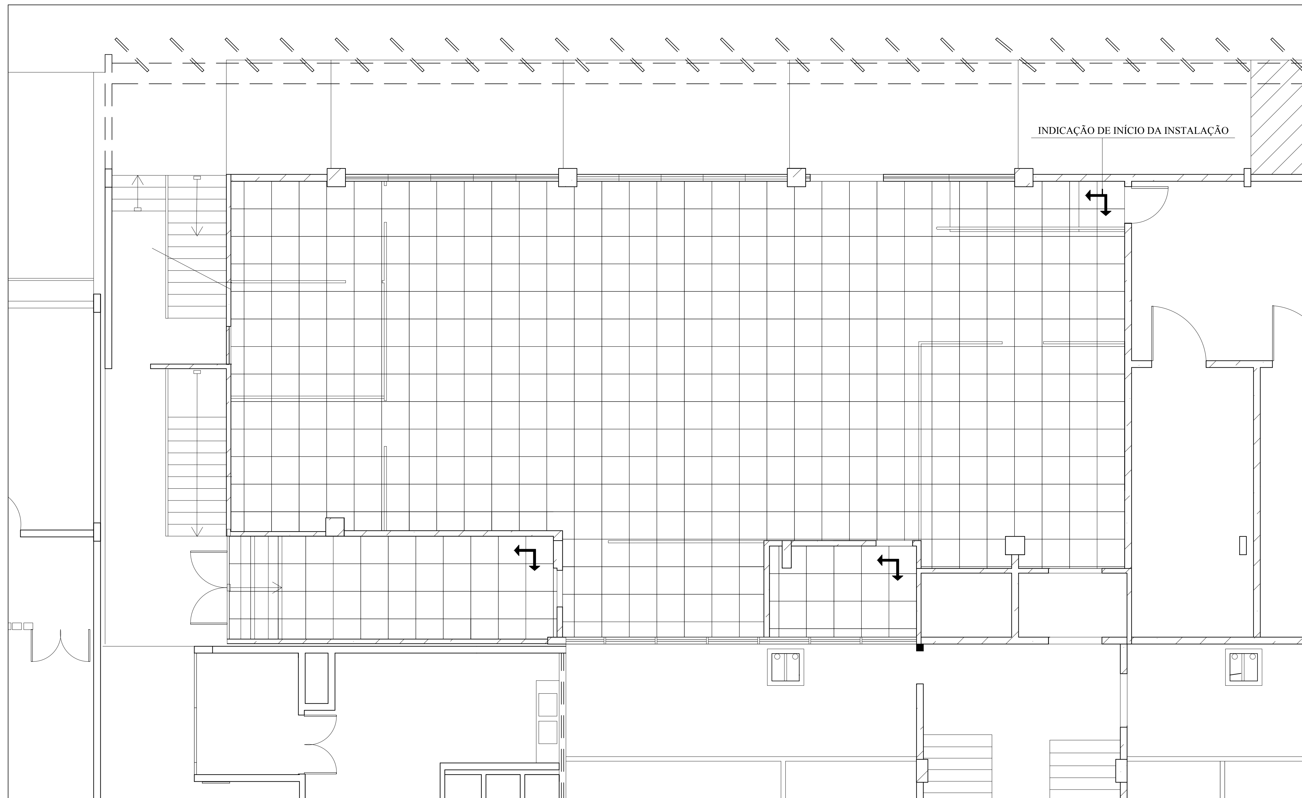
PLANTA DE PAGINAÇÃO DE FORRO ESCALA: 1/50
