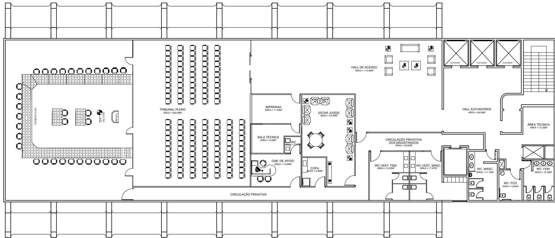
5º PAVIMENTO TIPO Esc.: 1/150
