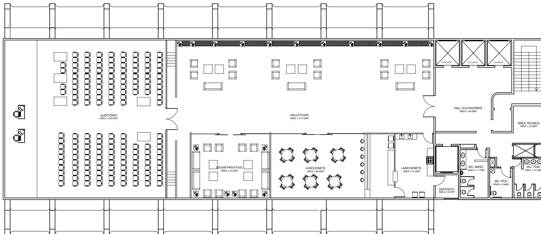
14º - PAVIMENTO TIPO Esc.: 1/150
